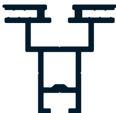
steckkederprofil 50/53 SEG frame 50/53
