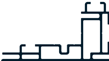
leuchtkastenprofil 100/55 light box profile 100/55
